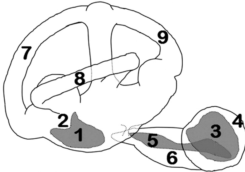
Figura 1. Estructura general de oído interno en Siluriformes. 1: lapillus , 2: utrículo , 3: asteriscus , 4: lagena , 5: sagitta , 6: sacculo , 7: canal antero-vertical, 8: canal horizontal, 9: canal posterior-vertical (extraído de Sánchez y Martínez 2017).
