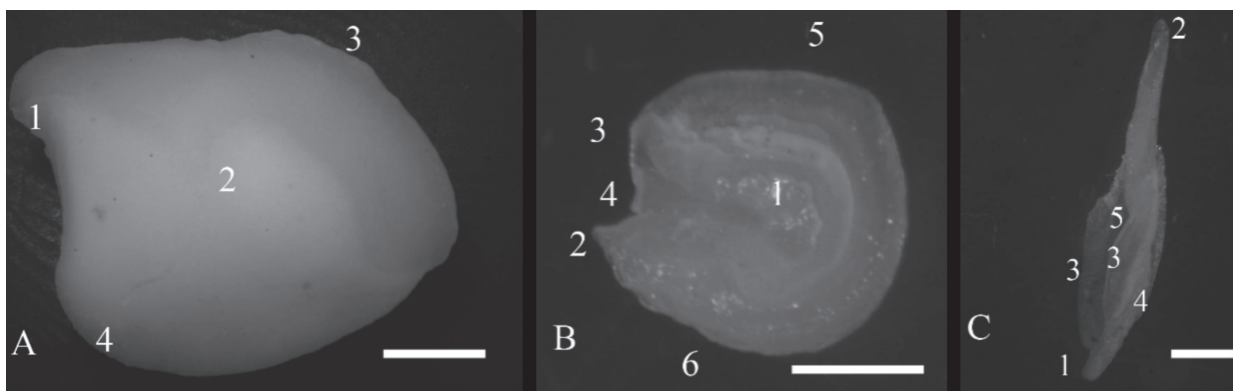
Figura 4. Estructura general y morfología de los tres tipos de otolitos de Genidens barbatus . A) Lapillus cara ventral, 1: sulcus, 2: elevación, 3: margen superior, 4: margen inferior. B) Asteriscus cara interna, 1: fosa acústica, 2: anti-rostrum, 3: rostrum, 4: excisión, 5: borde superior, 6: borde inferior. C) Sagitta cara interna, 1: región anterior, 2: región posterior, 3: alas dorsales, 4: ala basal, 5: fisura. Escala: 1,5 mm para lapillus , 0,25 mm para asteriscus y 0,5 mm para sagitta (adaptado de Sánchez y Martínez 2017).
